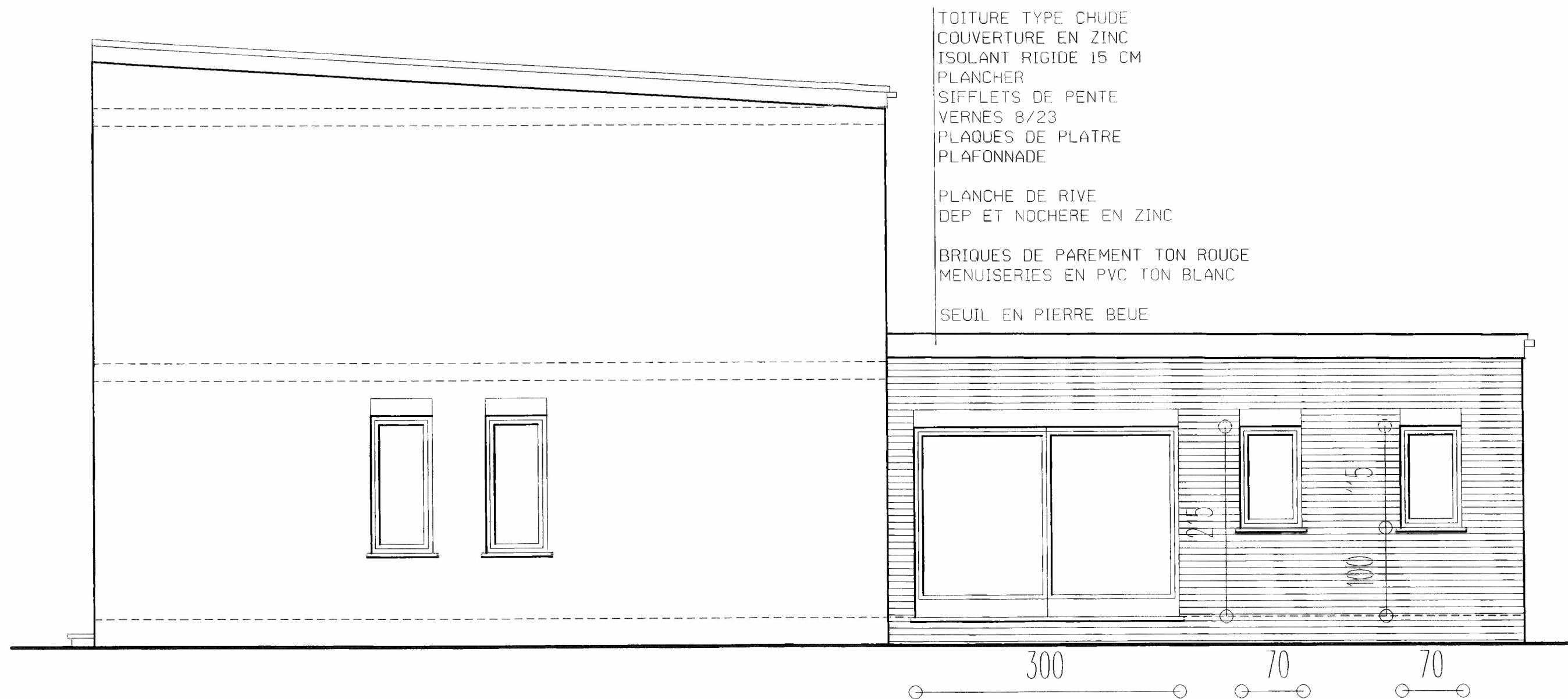
ELEVATION LATÉRALE DROITE
