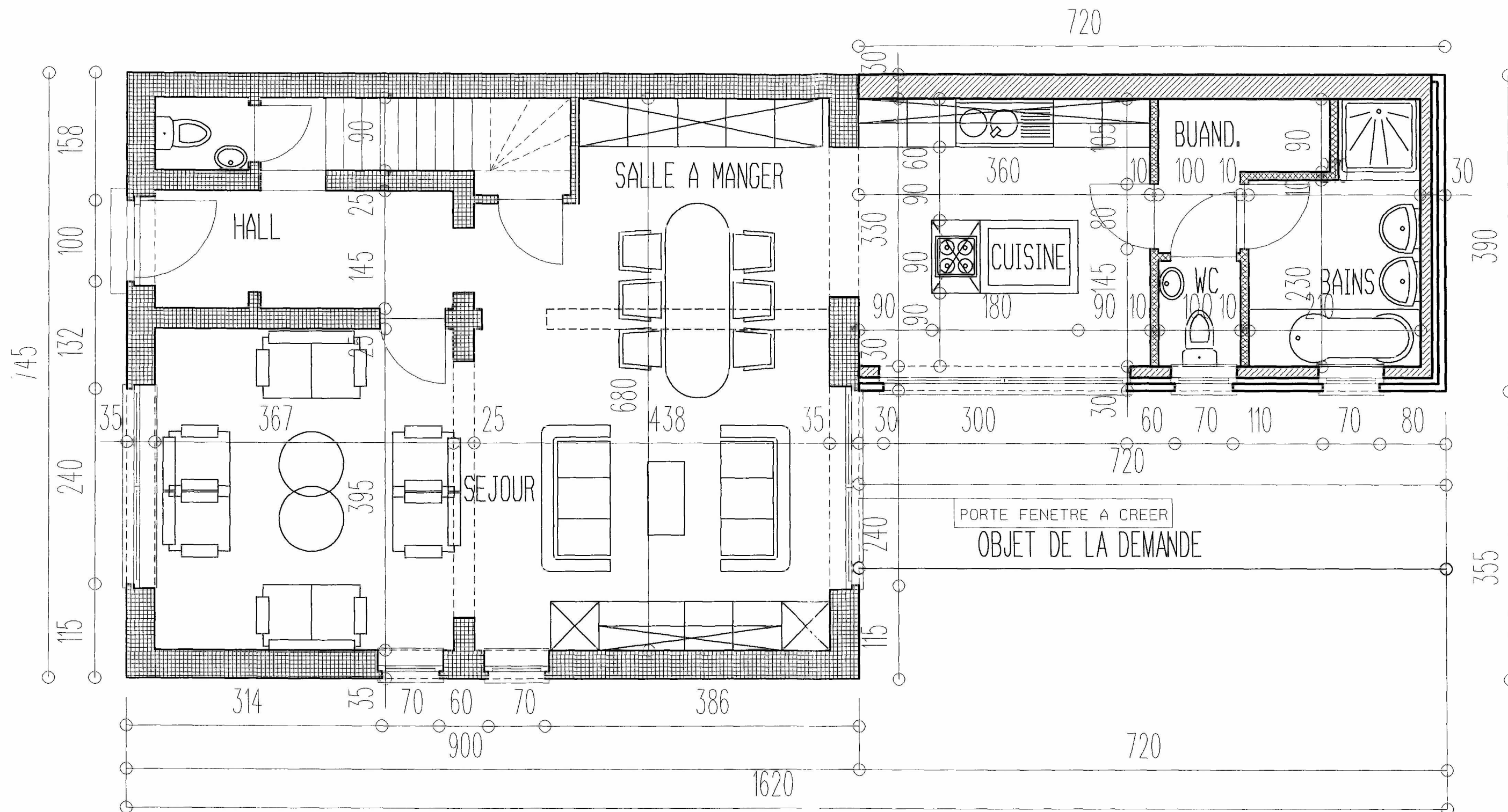
PLAN REZ DE CHAUSSEE
